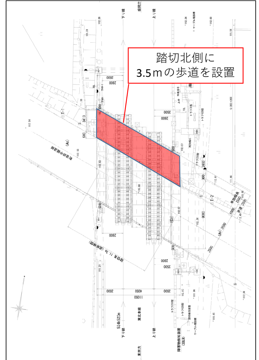
計画平面図
